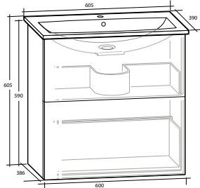
MÖBELPAKET 60 KOMPAKT, MED LÅDOR
