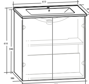
MÖBELPAKET 60 KOMPAKT, MED DÖRRAR
