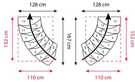
60° (12 × 5°)
