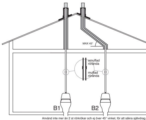
Använd inte mer än 2 st rörrökar och ej över 45° vinkel, för att säkra självdrag.
